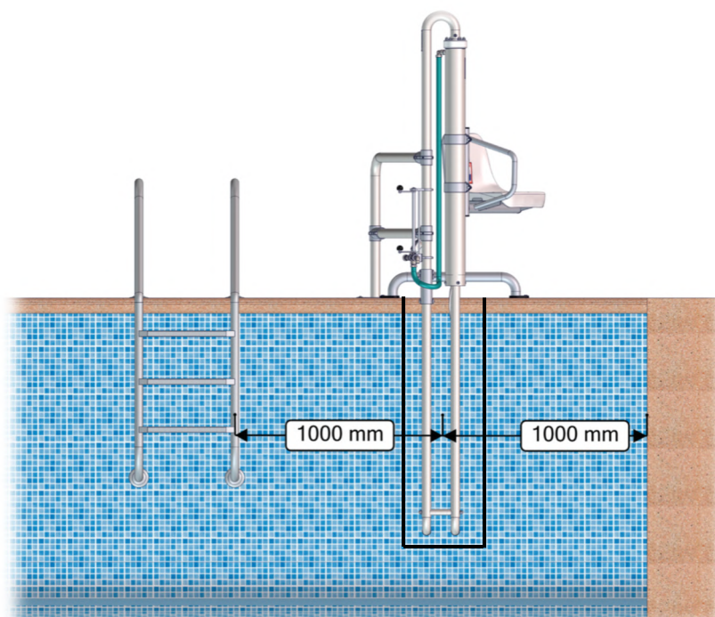
Espacio mínimo libre de obstáculos de 1 metro a cada lado.
